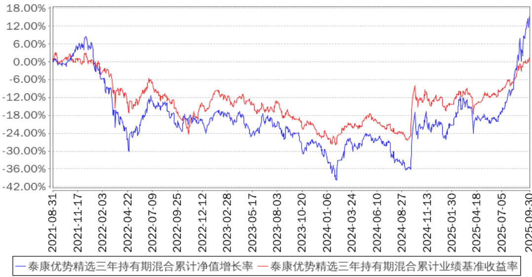
泰康优势精选三年持有期混合累计净值增长率与同期业绩比较基准收益率的历史走势对比图
